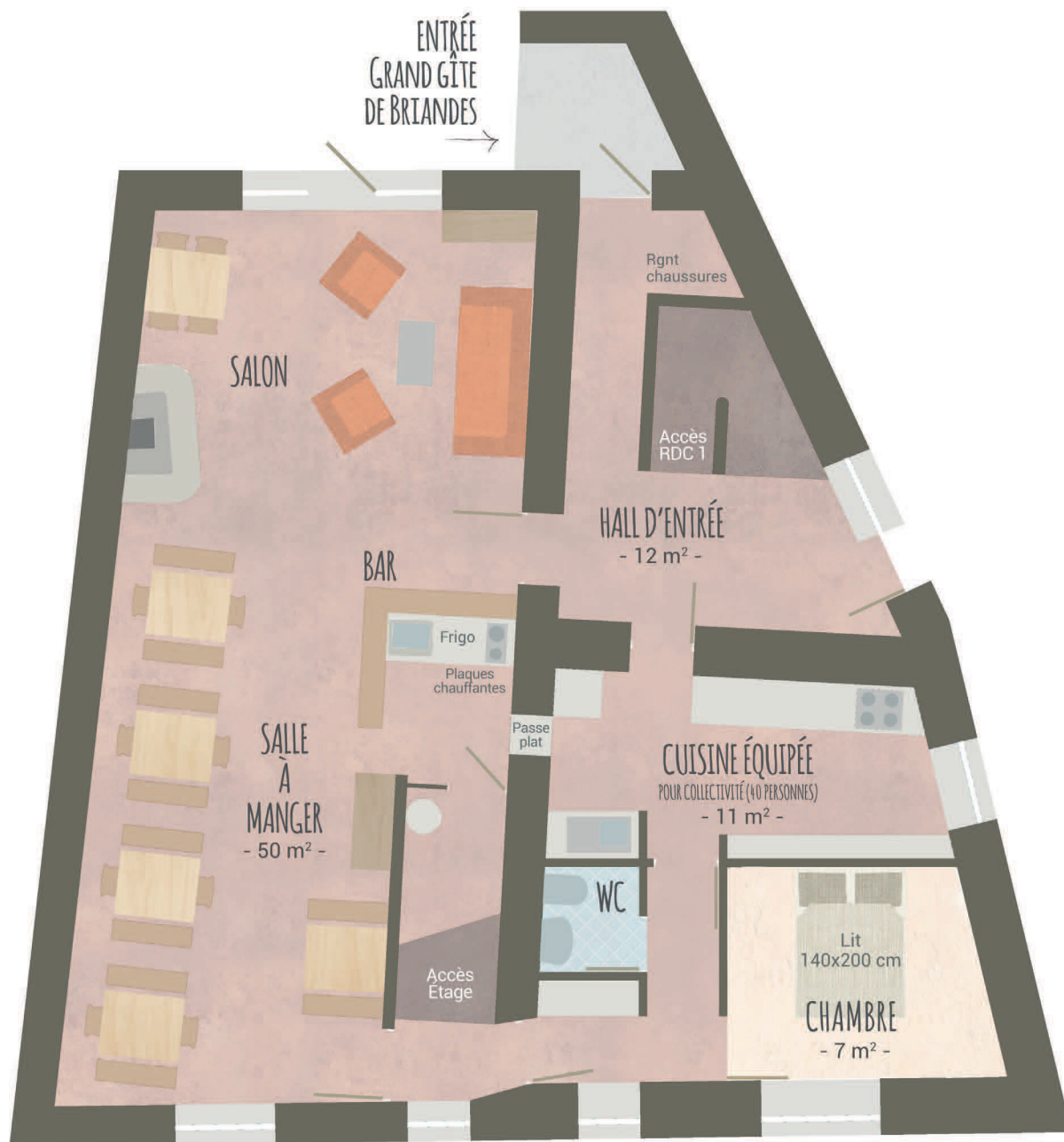
GRAND GÎTE DE BRIANDES - REZ DE CHAUSSÉE 2 -
